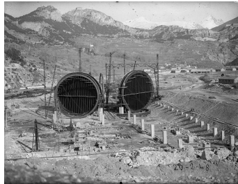
Construction de la Grande soufflerie de Modane
